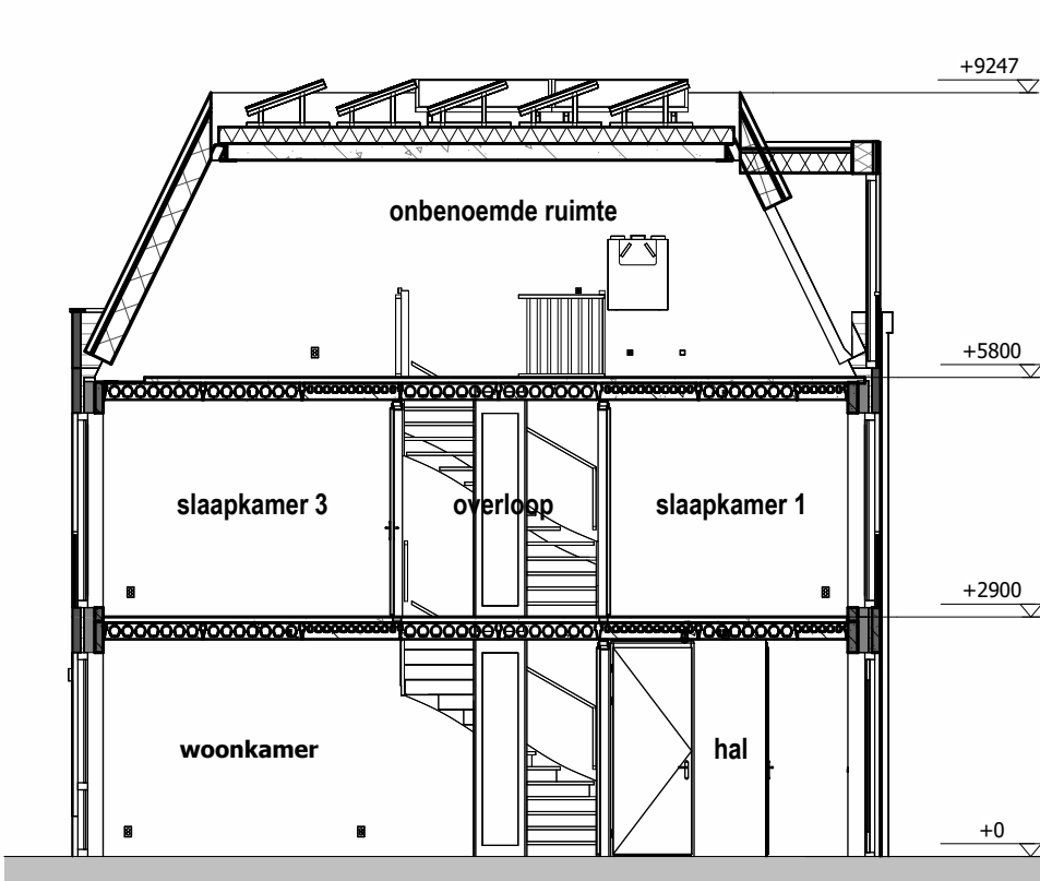
Doorsnede 1 : 100
